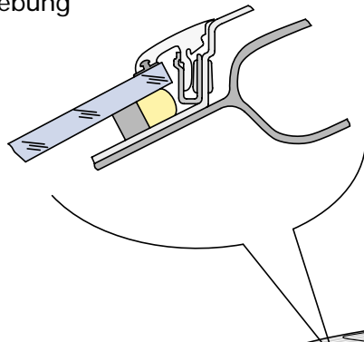
Windschutzscheiben- Verklebung
